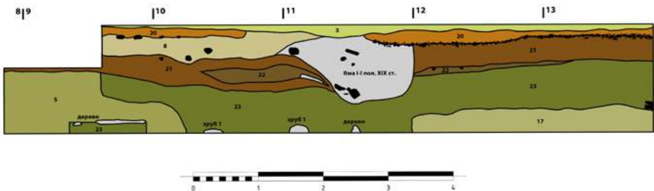
Рис. 7. Стратиграфія об'єкту № 2 по лінії b-b1 (рис. 4).
