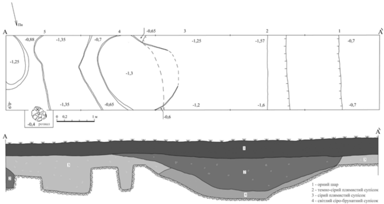
Рис. 4. План та стратиграфія рову. Троща 1, дослідження автора 2024 р.
