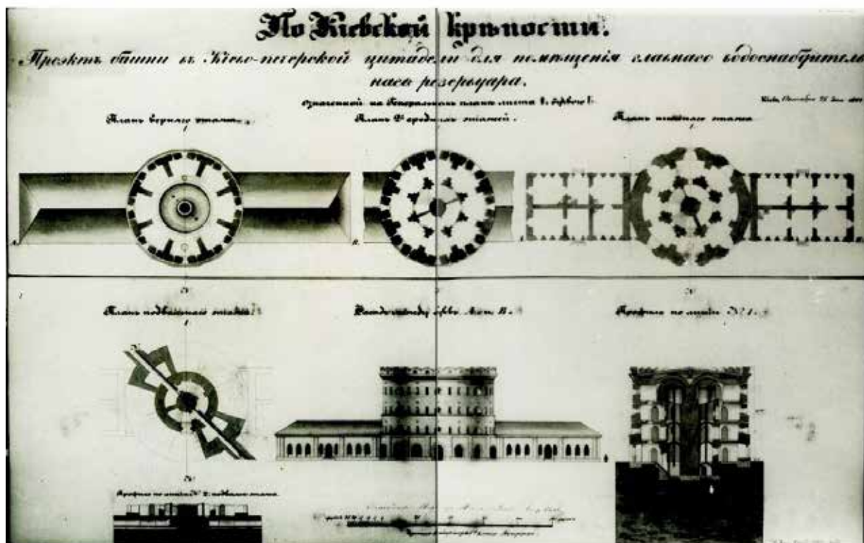
Рис. 6. План башни для розміщення головного резервуара з водою. Київська фортеця
