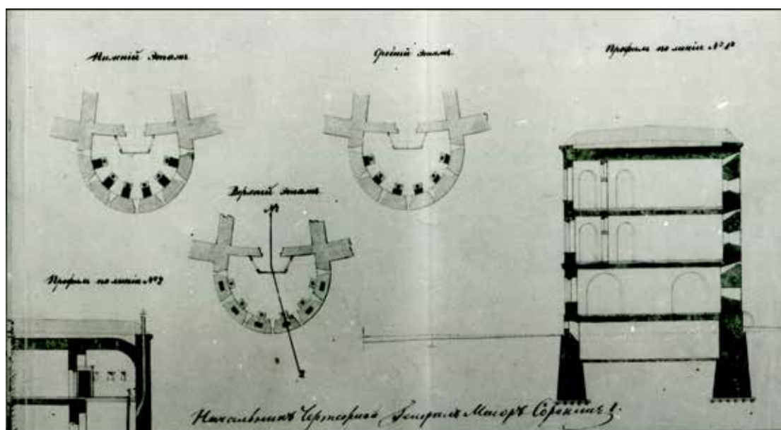
Рис. 5. План Басти № 8 Київської фортеці
