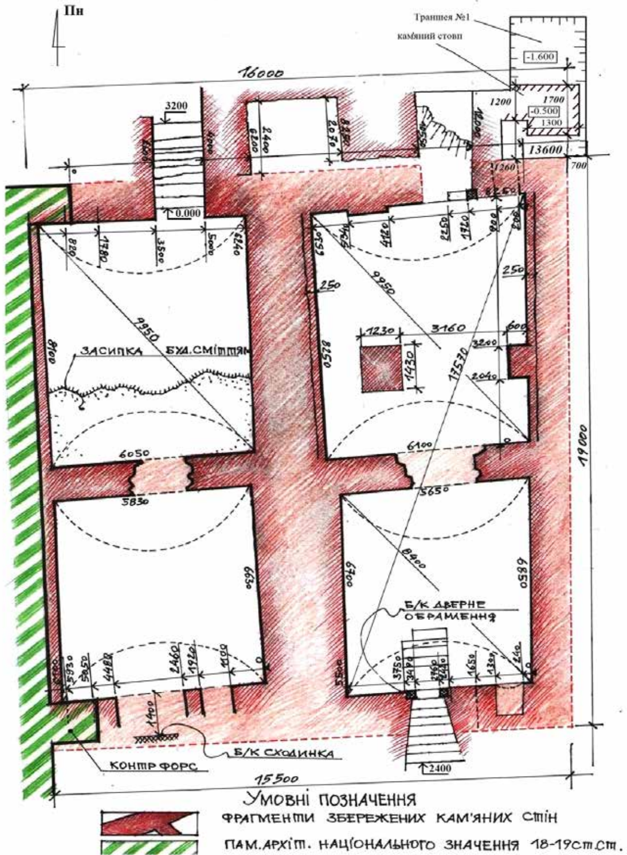
Рис. 3. План-схема фундаменту Вірменської ратуші (креслення – Л. І. Свінцицька)
