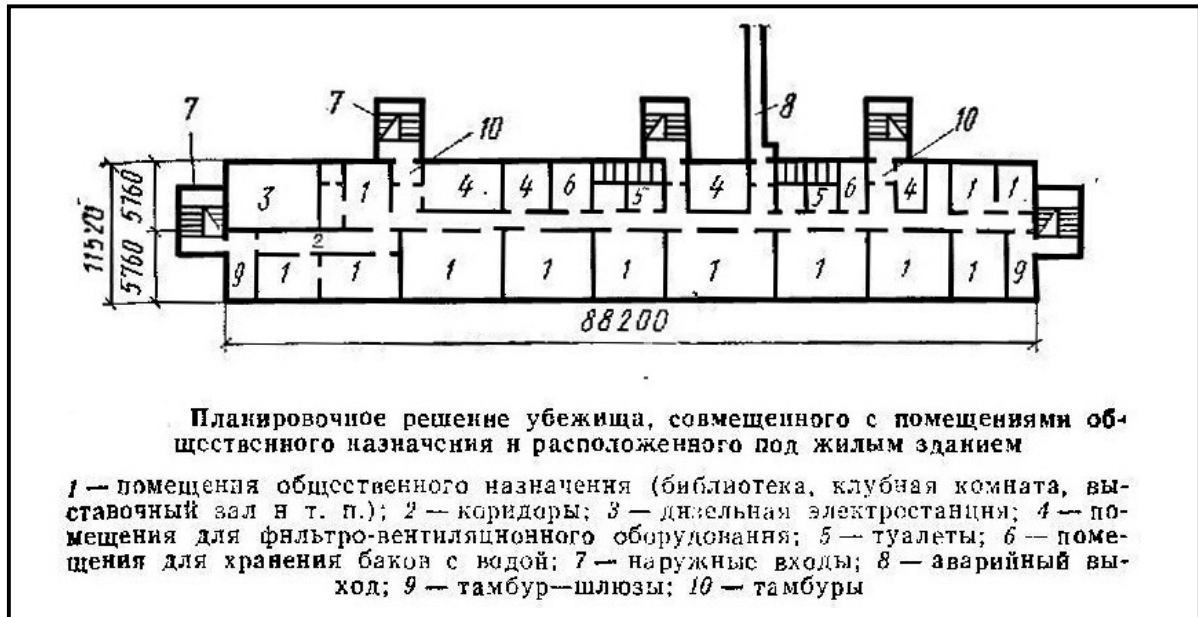
Рис. 3. Бомбосховище, поєднане із приміщеннями громадського призначення та розміщене під житловим будинком. Котляревський В.А. і др., Убежища гражданской обороны. Конструкции и расчет, Москва, Стройиздат, 1989, с. 135
