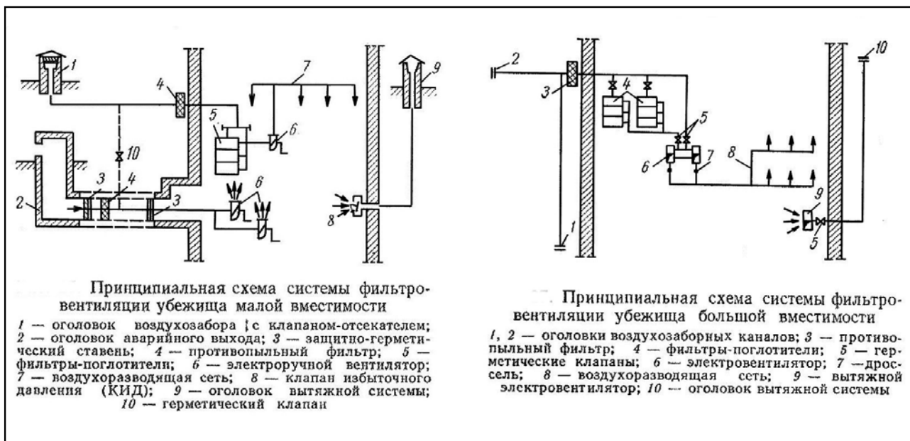
Рис.7 – Принципові схеми фільтро-вентиляції бомбосховищ малої та великої місткості. Зліва схема для сховища малої місткості, праворуч для сховища великої місткості. Камерер Ю.Ю., Харкевич А.Е., Експлуатація убежищ гражданской обороны, Москва, Стройиздат, 1970, с.58, 60
