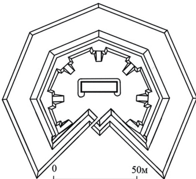
Рис. 1. План типового австрійського редути 1854–1855 років
