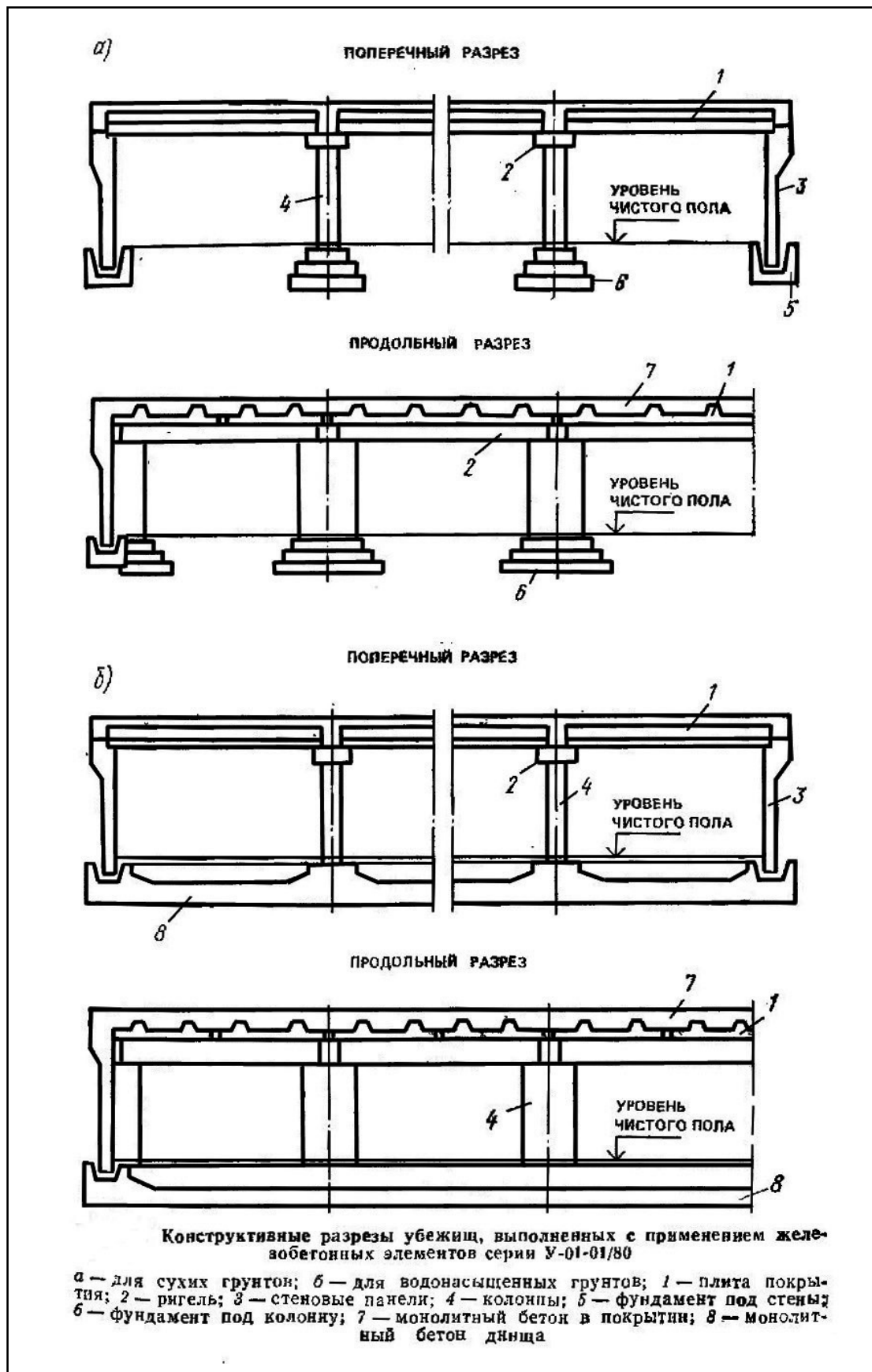
Рис. 5. Переріз бомбосховищ, виконаних із застосуванням типових залізобетонних елементів серії У-01-01/80, розроблених для зведення захисних споруд. Котляревський В.А. і др., Убежища гражданской обороны. Конструкции и расчет, Москва, Стройиздат, 1989, с. 139
