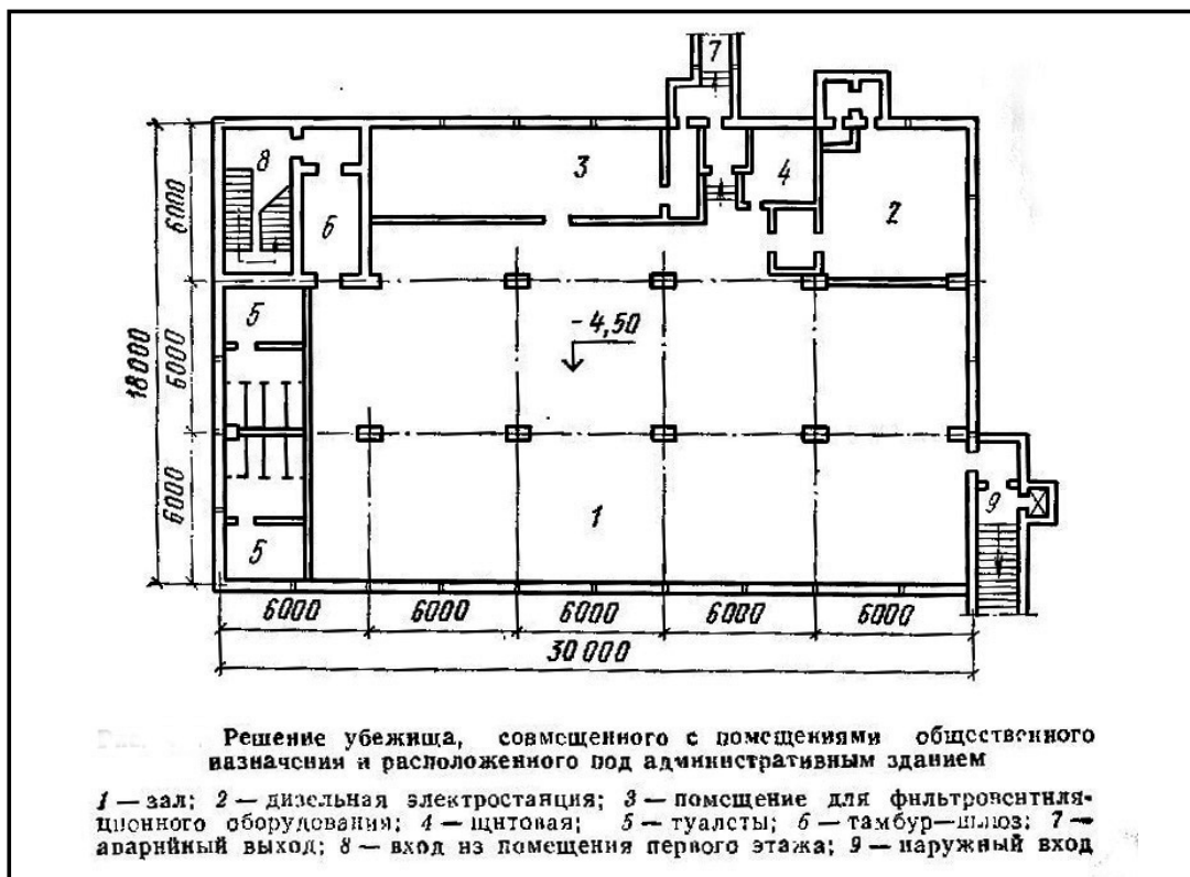
Рис. 2. Бомбосховище, поєднане із приміщенням громадського призначення та розміщене під адміністративним будинком. Котляревский В.А. и др., Убежища гражданской обороны. Конструкции и расчет, Москва, Стройиздат, 1989, с. 134
