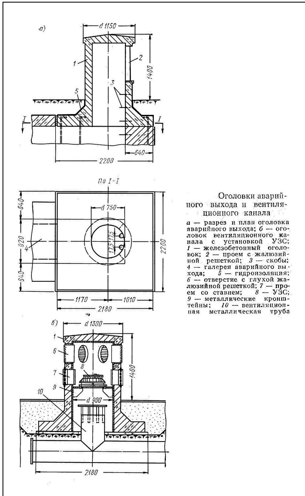
Рис. 6. Оголовки аварийного выхода та вентиляційного каналу. Камерер Ю.Ю., Харкевич А.Е., Эксплуатация убежищ гражданской обороны, Москва, Стройиздат, 1970, с. 12
