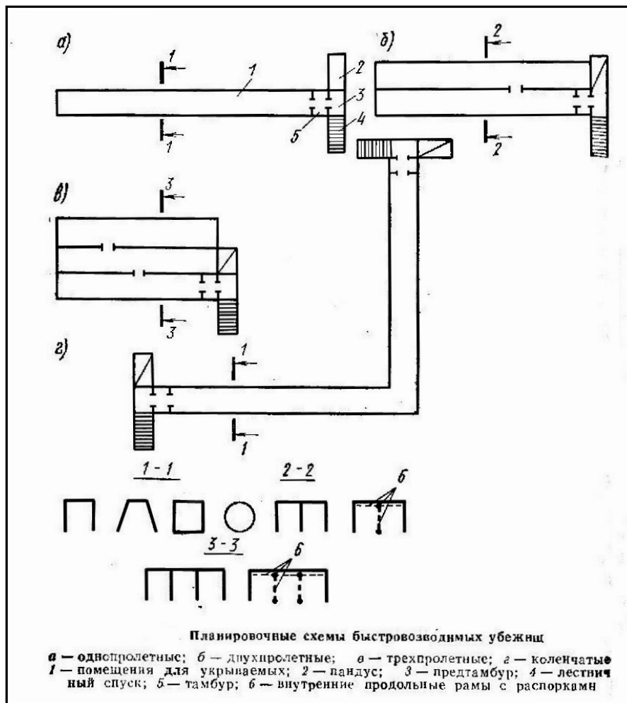
Рис. 4. Схеми та перерізи бомбосховищ, що швидко зводяться в загрожуваній період. Котляревський В.А. і др., Убежища гражданской обороны. Конструкции и расчет, Москва, Стройиздат, 1989, с. 172
