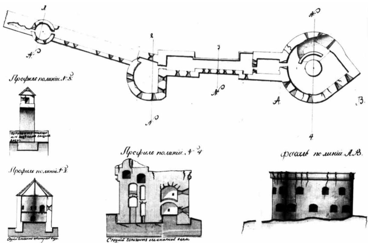
Рис. 1. План, фасад та розріз Прибережної башти за креслеником 1800 р.
