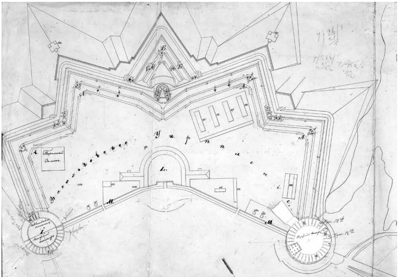
Рис. 1. Васильківське укріплення. Джерело: ЦДІАК України, ф. 1434, оп. 1, сп. 2, л. 9
