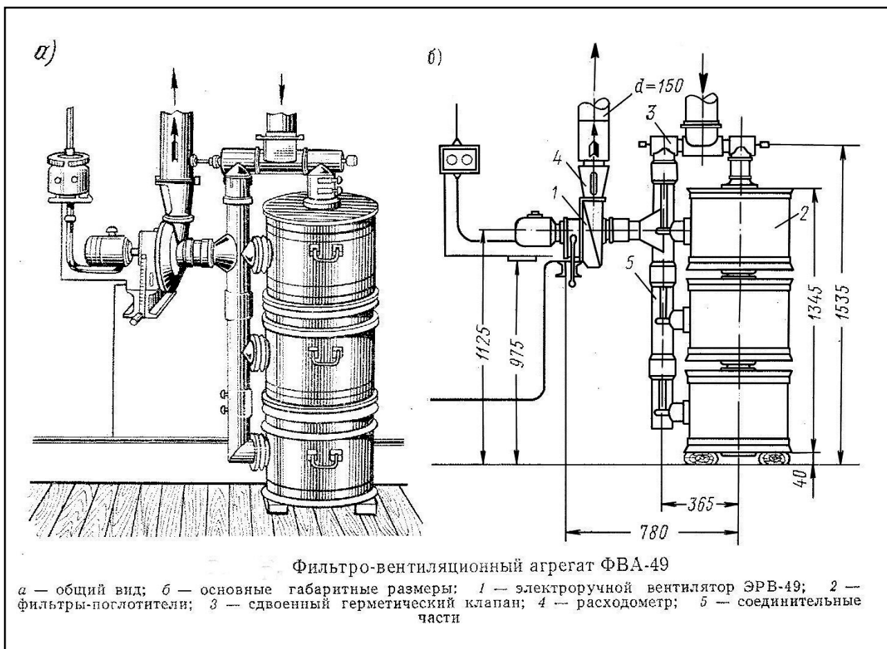
Рис. 8. Фільтровентиляційний агрегат ФВА-49. Камерер Ю.Ю., Харкевич А.Е., Експлуатація убежищ гражданской обороны, Москва, Стройиздат, 1970, с. 59
