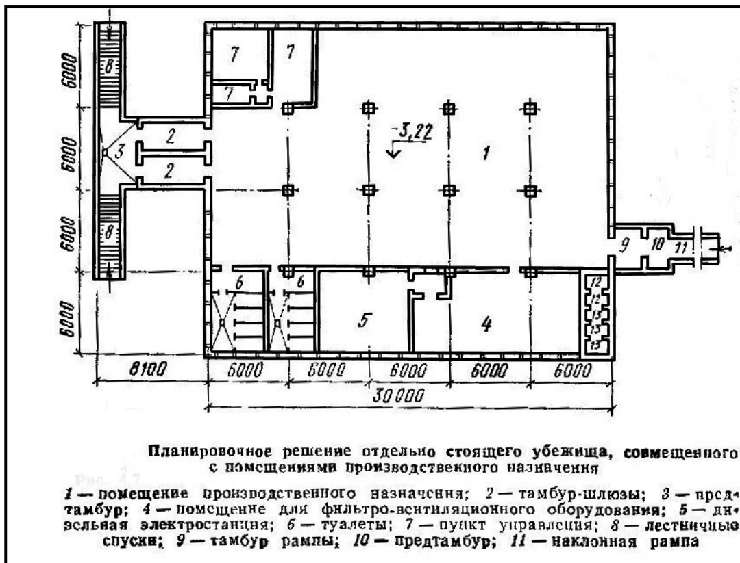
Рис. 1. Планування окремо розташованого бомбосховища, поєднаного з приміщенням виробничого призначення. Котляревский В.А. и др., Убежища гражданской обороны. Конструкции и расчет, Москва, Стройиздат, 1989, с. 134
